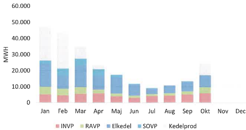
Figur 3 Produktionsfordeling pr. måned i MW
