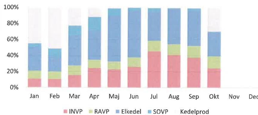
Figur 2 Produktionsfordeling pr. måned i procent
